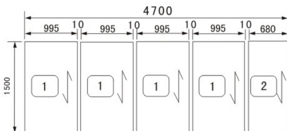
钢格板排版图
